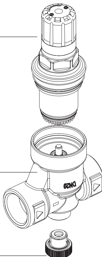
Druckmindererpatrone
