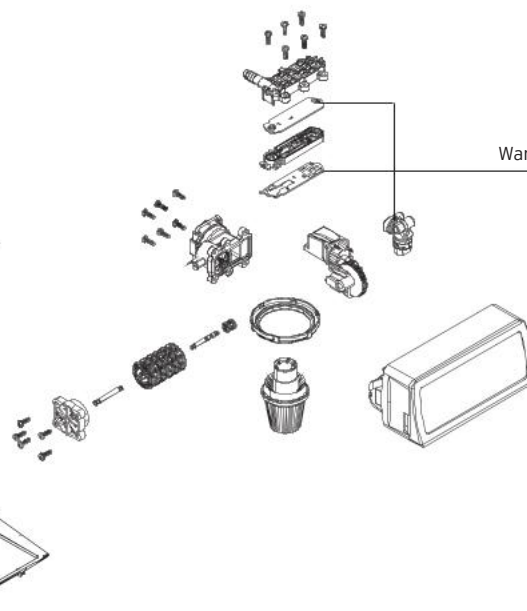
Steuerkopf
