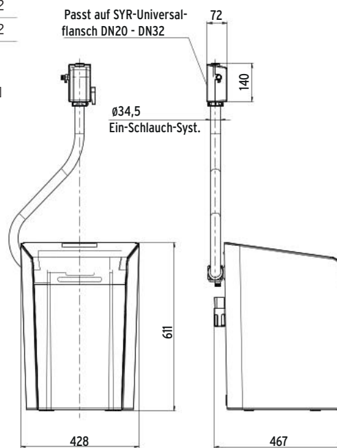
Dreifach-Trichtersiphon Maße [mm]
